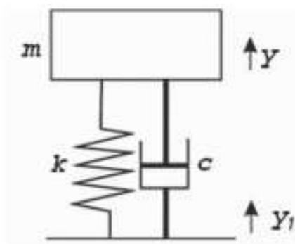
1.6 – rasm. Avtomobilning kotarib turuvchi sistemasining sxemasi
