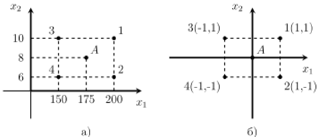
3.1-rasm. 2^2 to'liq faktorli eksperimentning eksperimental nuqtalarining joylashuvi
