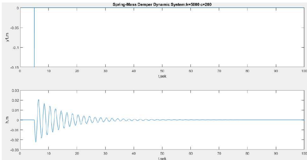
1.13-rasm. Modelning ishlash natijasi
