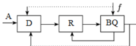
1-rasm. Optimal boshqarish tizimi umumiy blok-sxemasi.
